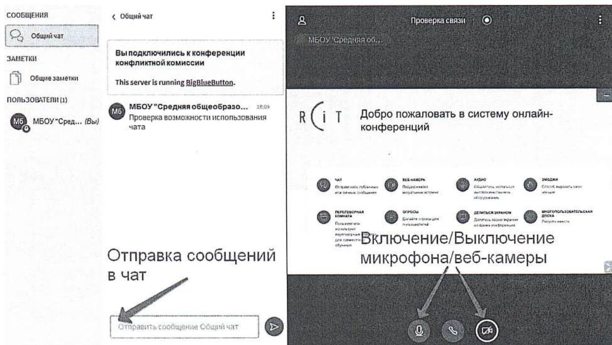
Рисунок 6 – Интерфейс ИС
