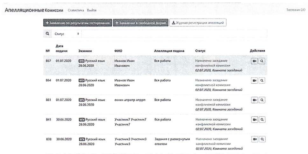
Рисунок 3 - Интерфейс ИС
